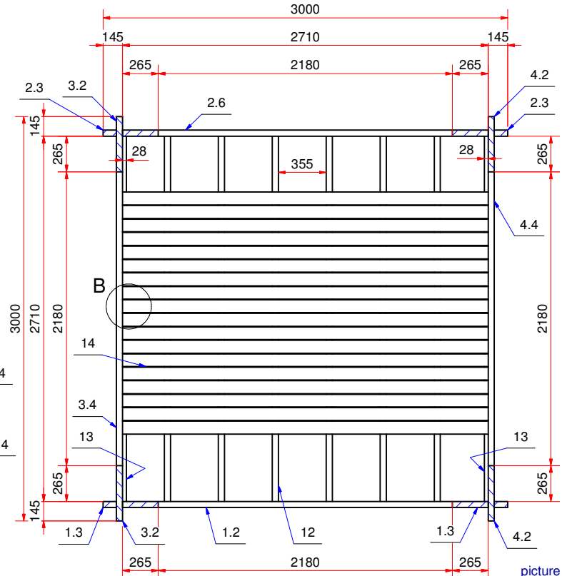
План дома (house plan)
