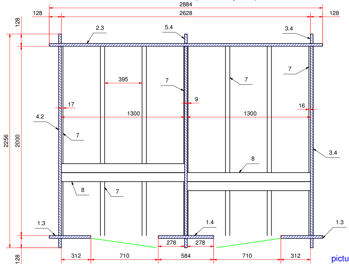
План дома (house plan)
