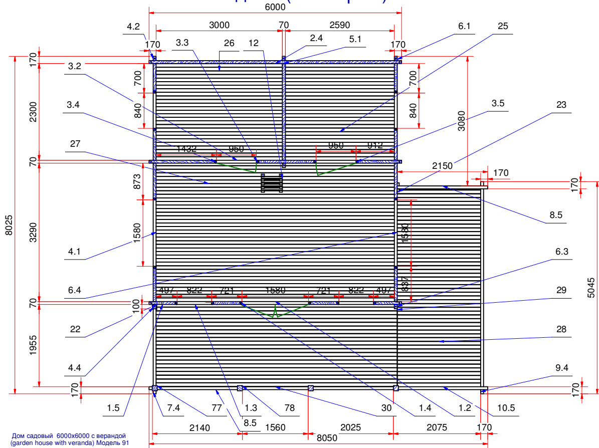
План дома (house plan)
