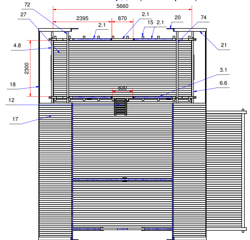
План мансарды (house plan)
