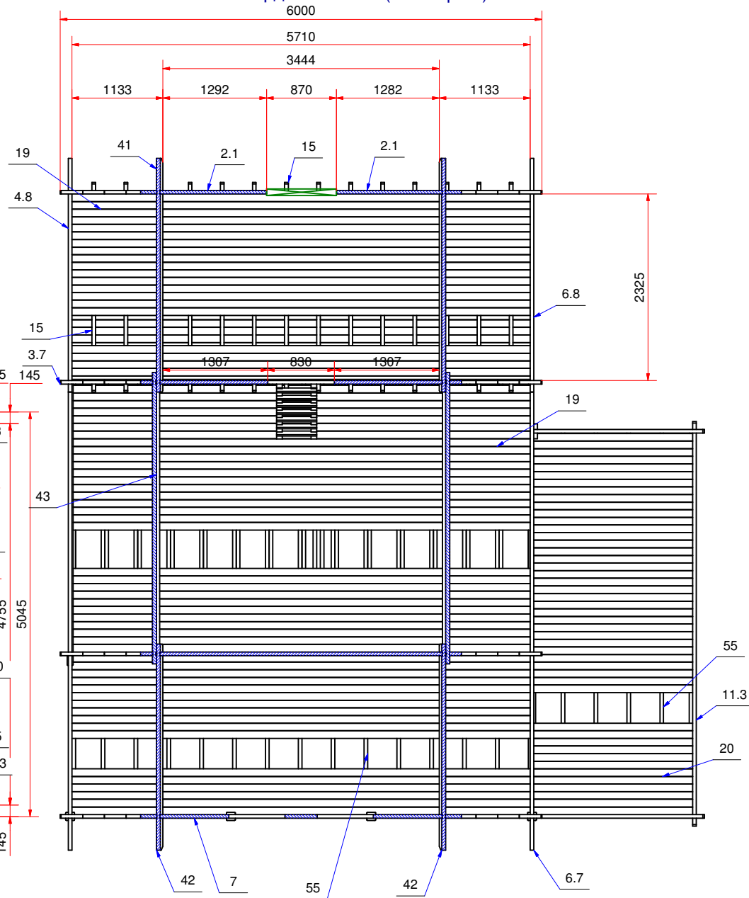
План мансардного этажа (house plan)
