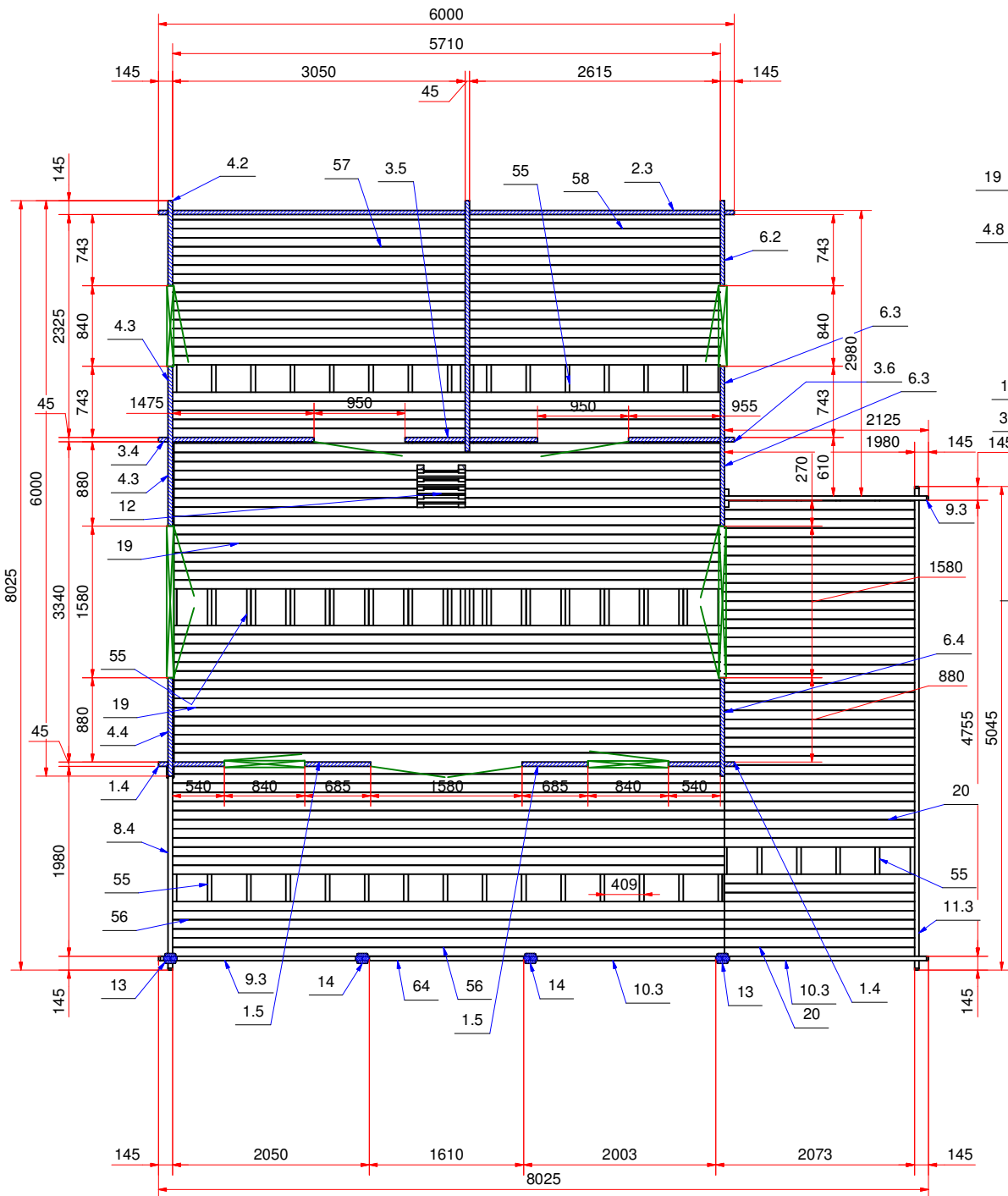
План дома (house plan)
