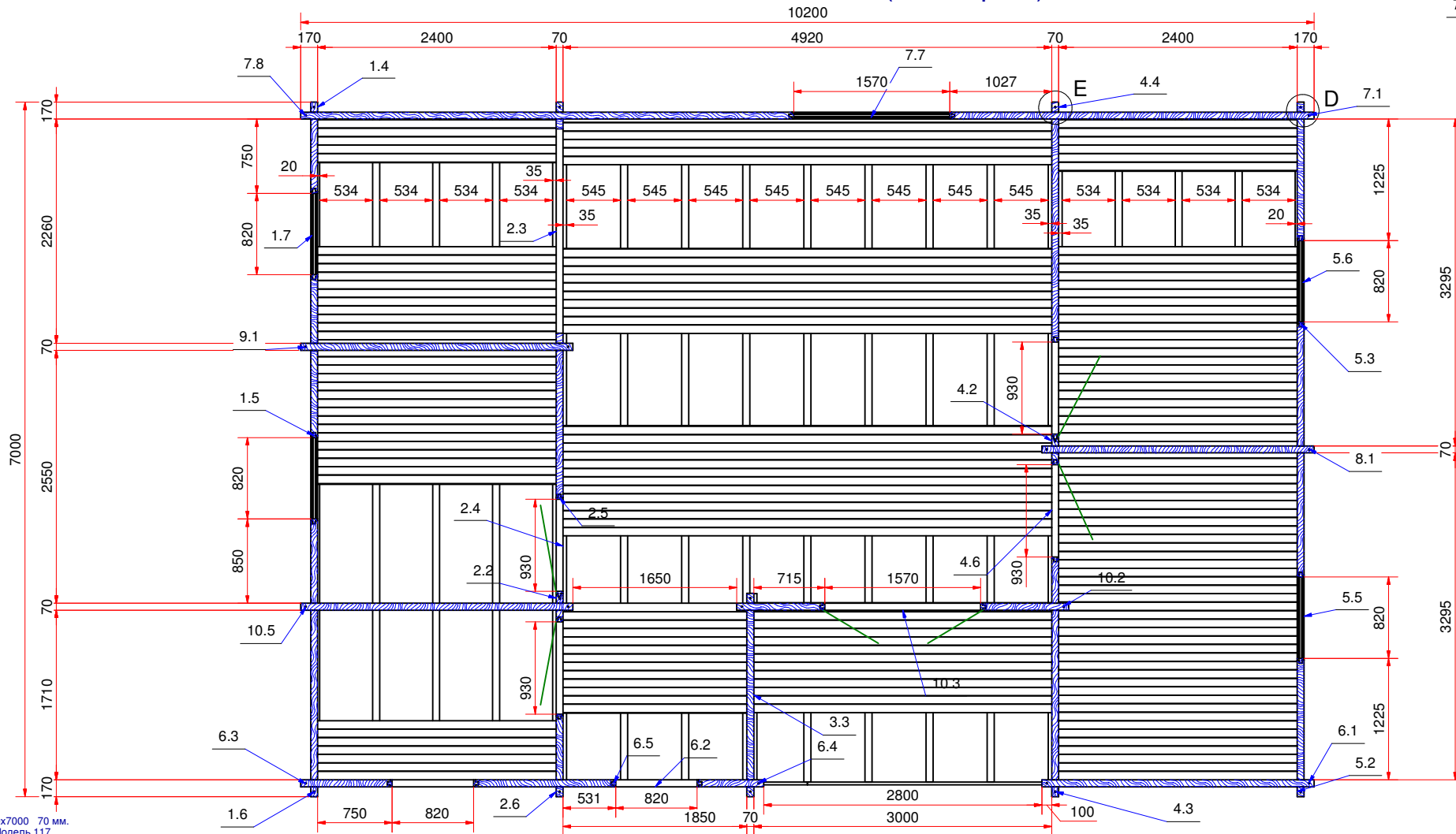
План дома (house plan)
